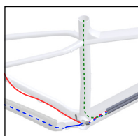
Vedení bowdenů a hadiček - teleskopická sedlovka, bez přesmykače
